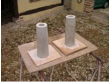
Tuyère mono cylindrique
